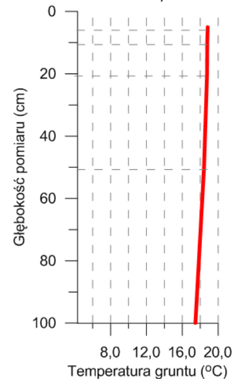
Średnia miesięczna temperatura gruntu Borucino - sierpień 2019
