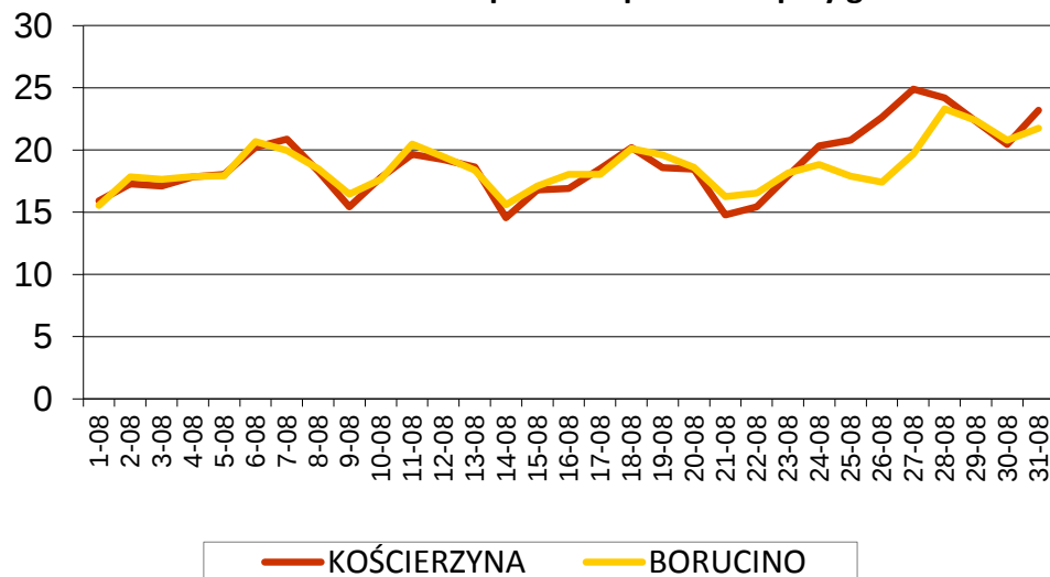
Średnia dobową temperaturę powietrza przy gruncie
