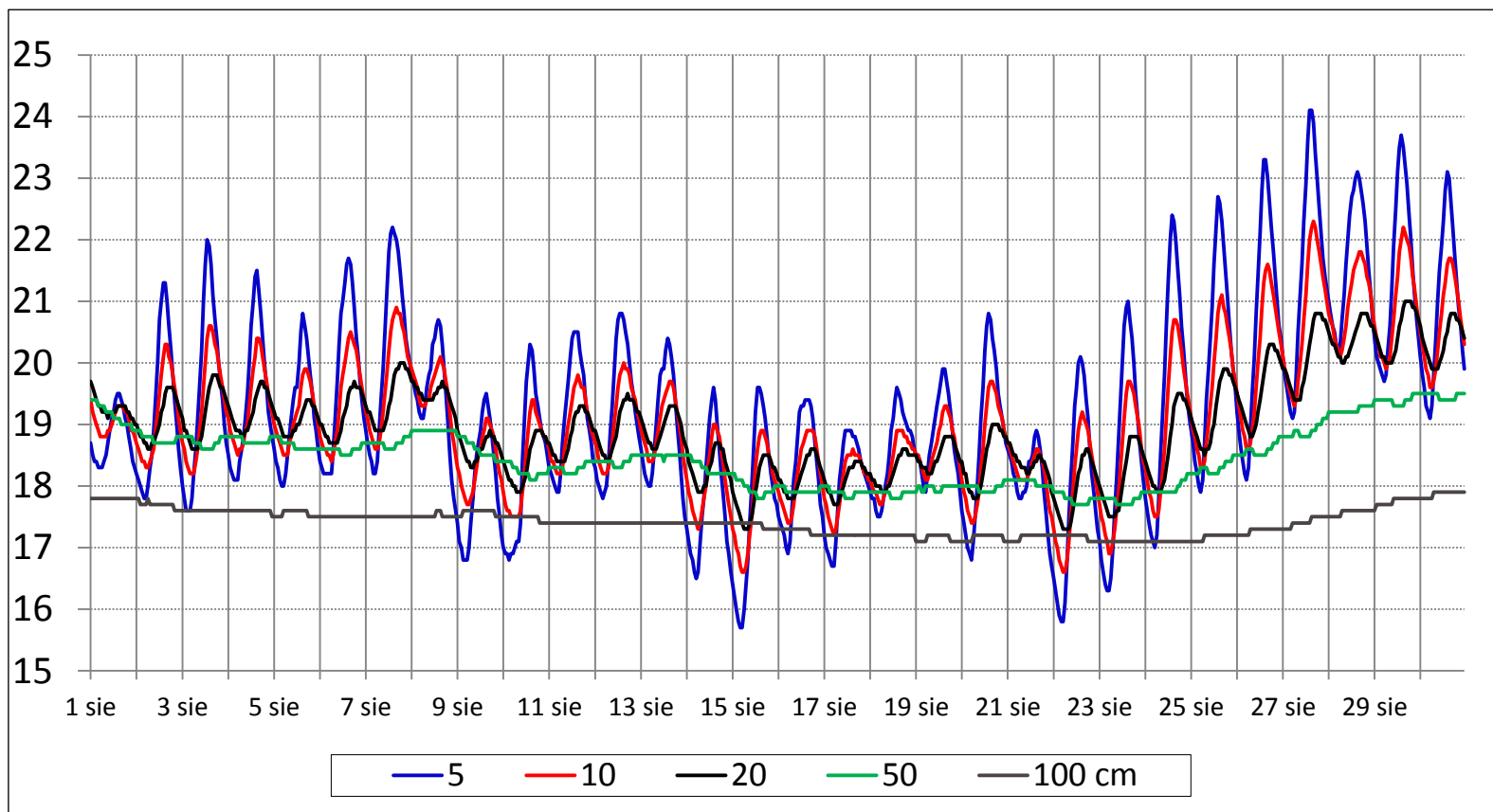
Średnia miesięczna temperatura gruntu Borucino - sierpień 2019
