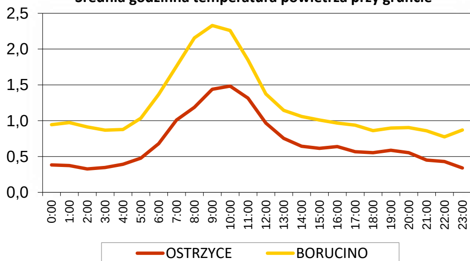
Średnia godzinna temperatura powietrza przy gruncie
