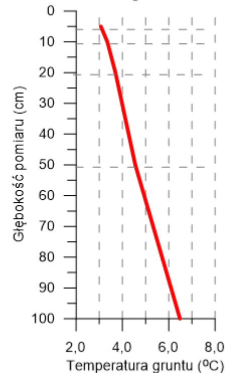
Średnia miesięczna temperatura gruntu Borucino - grudzień 2020
