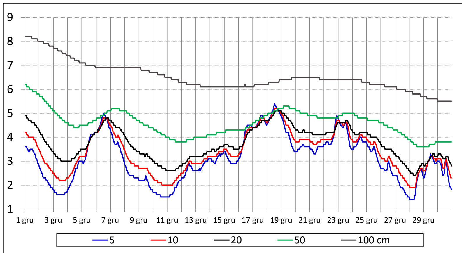
Średnia miesięczna temperatura gruntu Borucino - grudzień 2020
