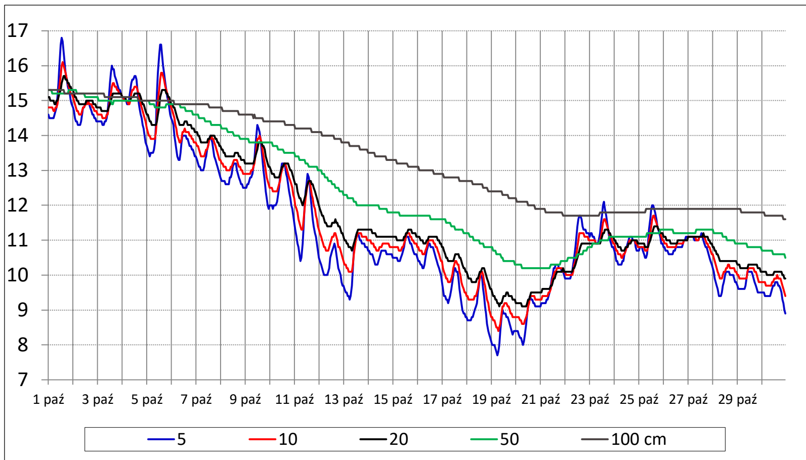
Średnia miesięczna temperatura gruntu Borucino - październik 2020
