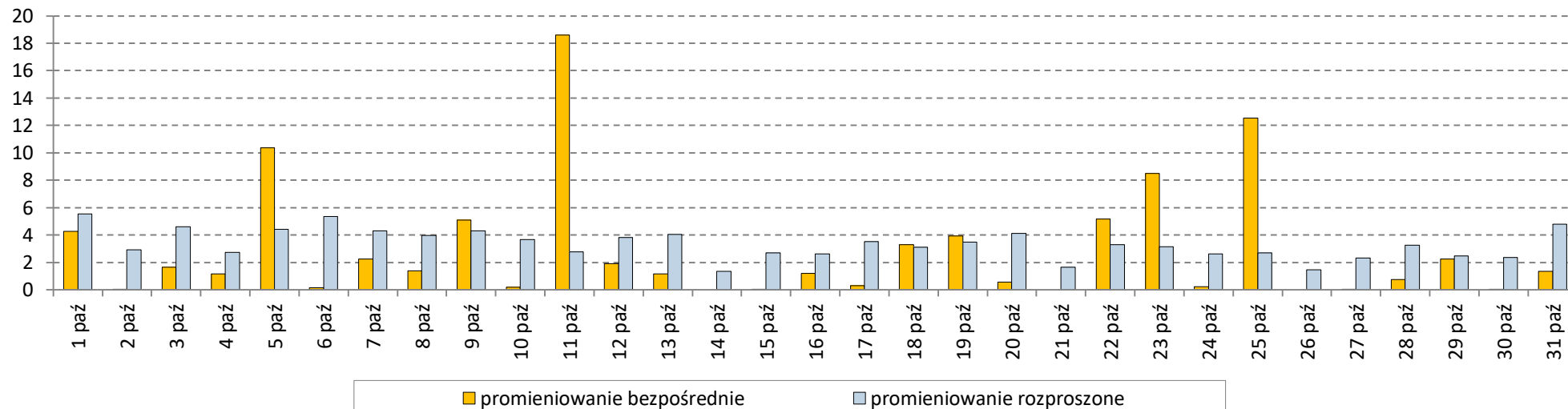
Sumy dobowe energii promieniowania bezpośredniego i rozproszonego [ \text{MJ} \cdot \text{m}^{-2} ]
