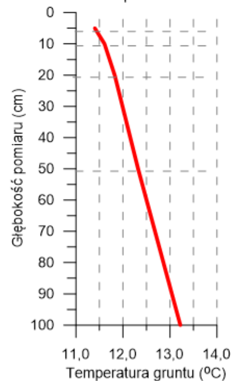
Średnia miesięczna temperatura gruntu Borucino - październik 2020
