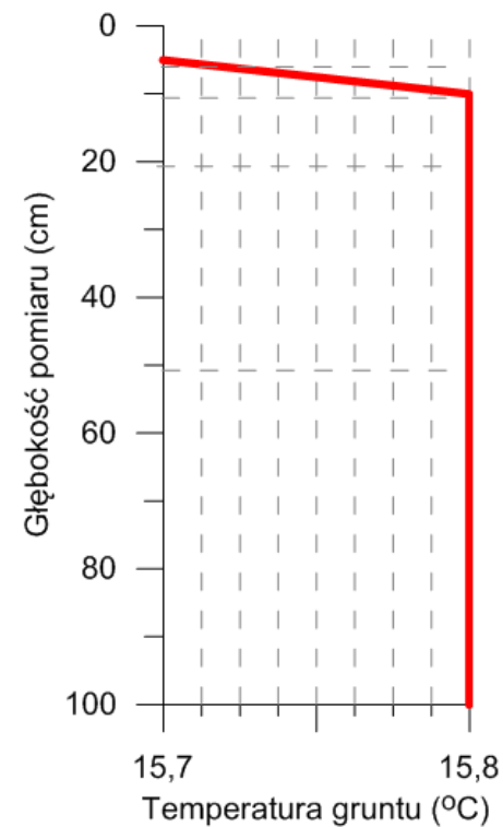
Średnia miesięczna temperatura gruntu Borucino - wrzesień 2020
