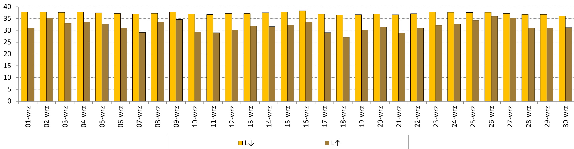
Sumy dobowe energii promieniowania długofalowego [ \text{MJ}\cdot\text{m}^{-2} ]
