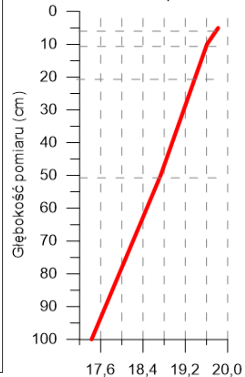
Średnia miesięczna temperatura gruntu Borucino - sierpień 2020
