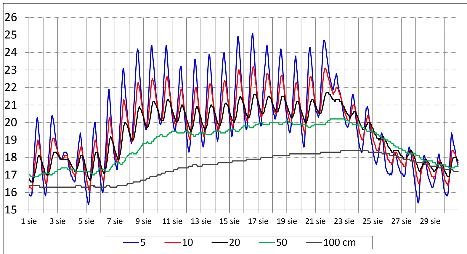
Średnia miesięczna temperatura gruntu Borucino - sierpień 2020
