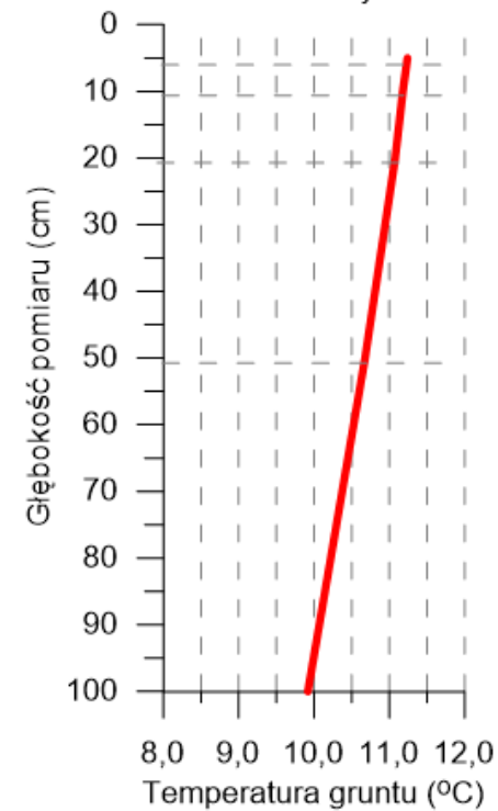
Średnia miesięczna temperatura gruntu Borucino - maj 2020
