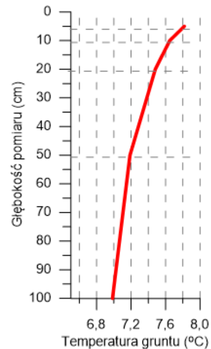
Średnia miesięczna temperatura gruntu Borucino - kwiecień 2020
