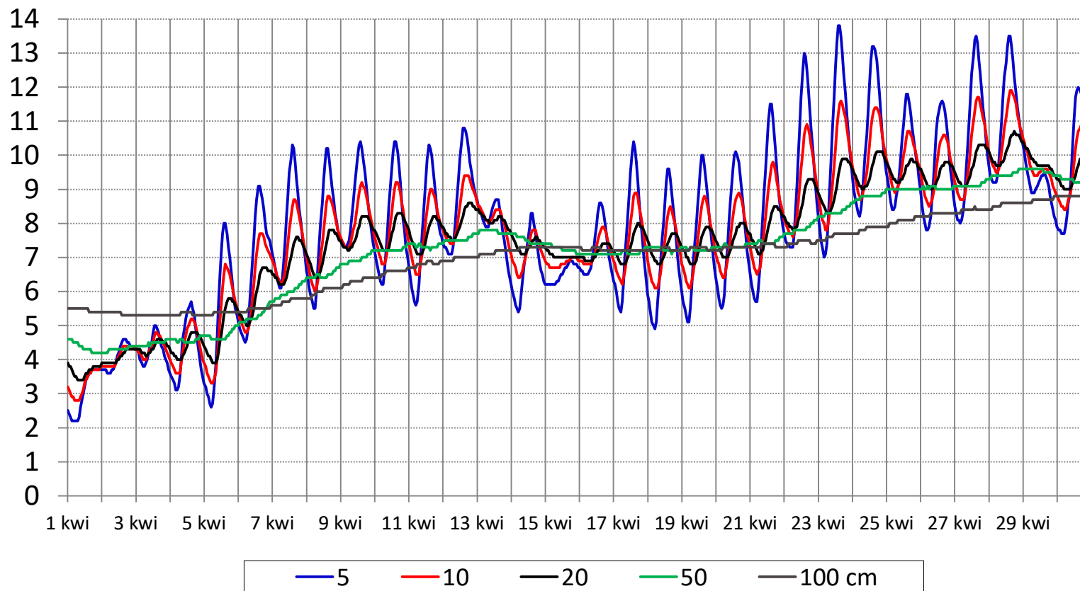
Średnia miesięczna temperatura gruntu Borucino - kwiecień 2020
