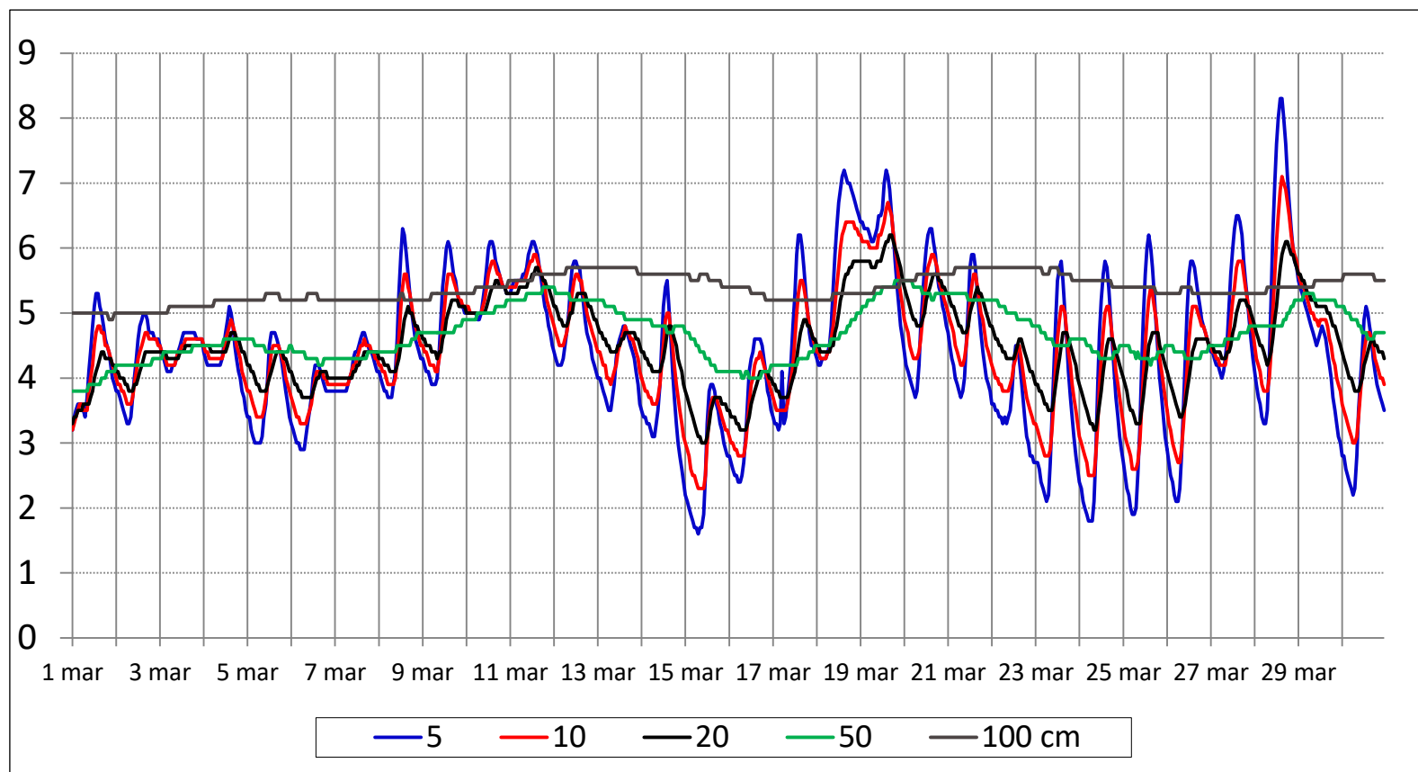
Średnia miesięczna temperatura gruntu Borucino - marzec 2020
