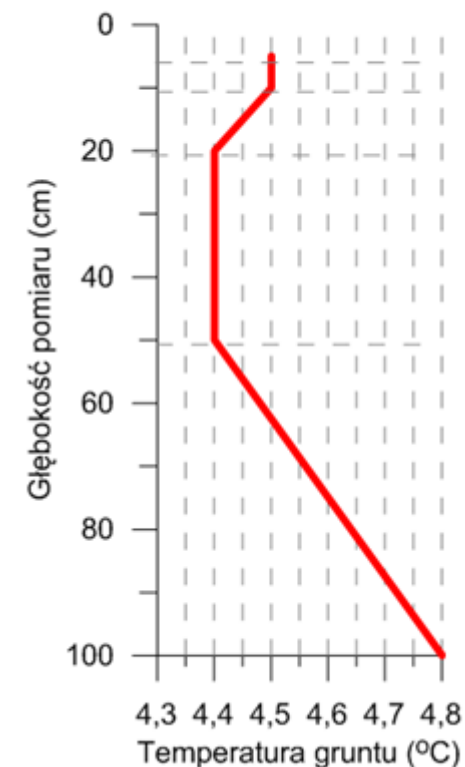
Średnia miesięczna temperatura gruntu Borucino - marzec 2020
