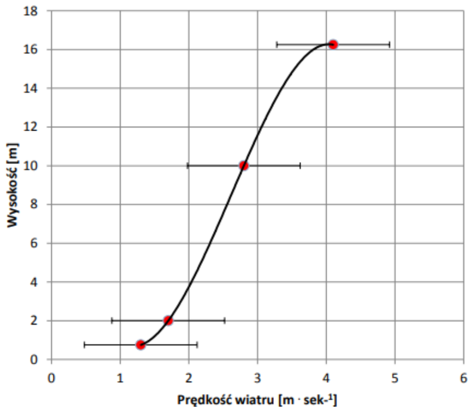
Zmienność średniej miesięcznej prędkości wiatru wraz z wysokością
