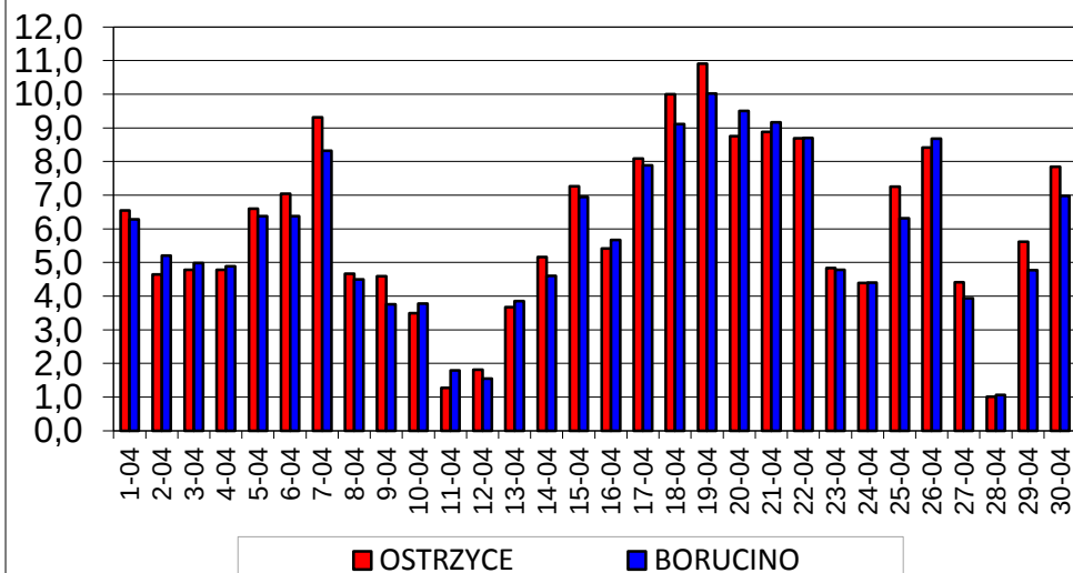
Temperatura przy gruncie - odchylenie standardowe [°C]
