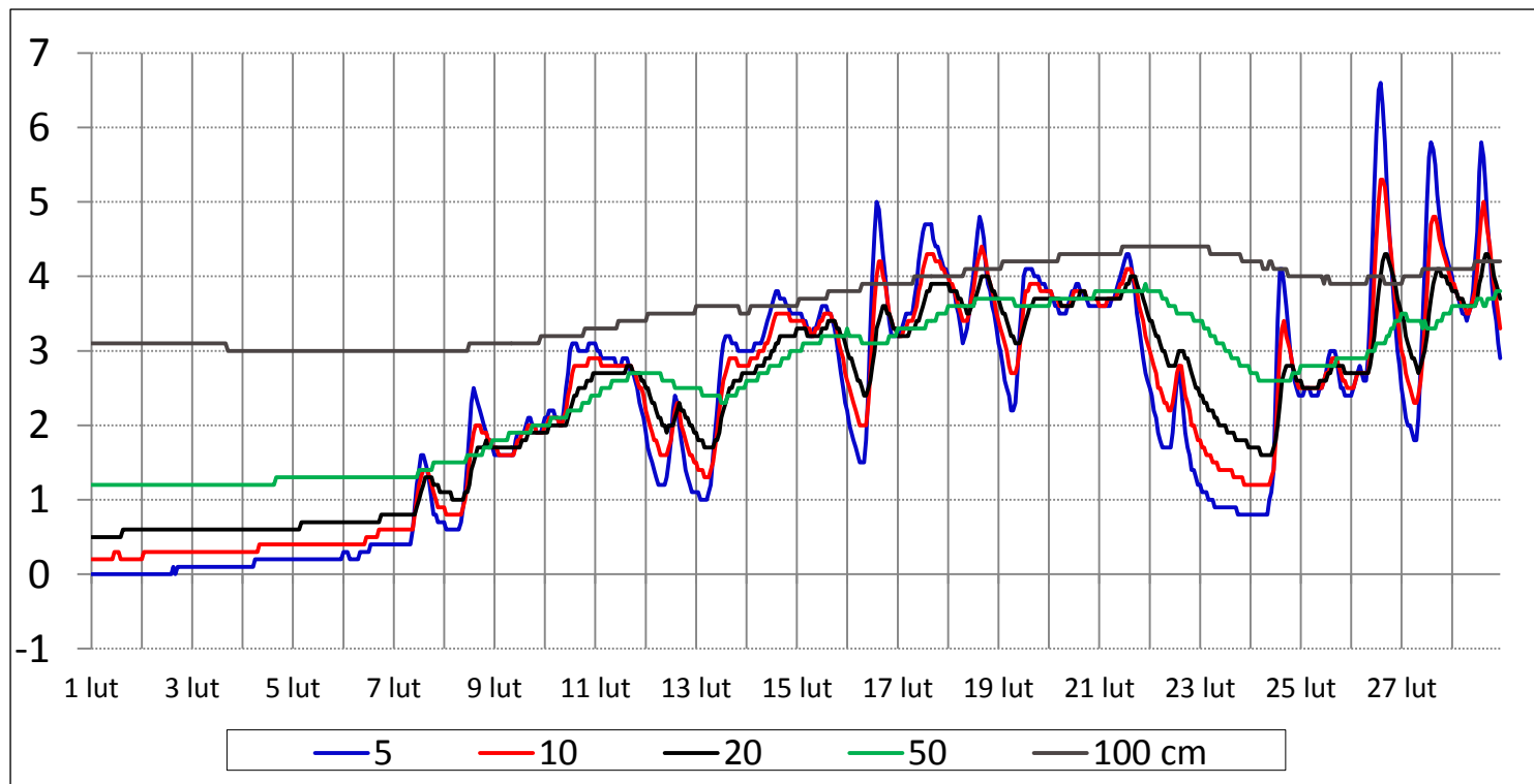
Średnia miesięczna temperatura gruntu Borucino - luty 2019
