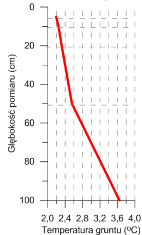
Średnia miesięczna temperatura gruntu Borucino - luty 2019
