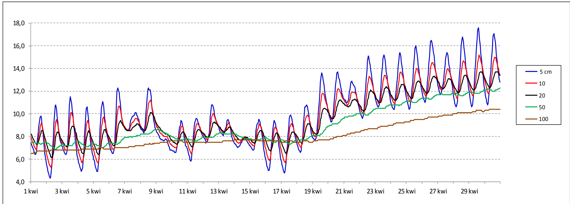
Średnia miesięczna temperatura gruntu Borucino - kwiecień 2014
